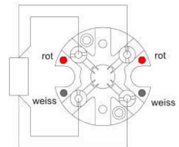
1xPt100 4-Leiter
