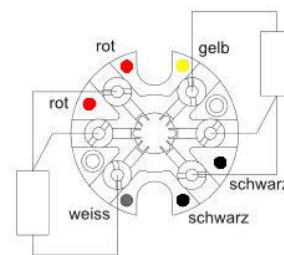
2xPt100 3-Leiter
