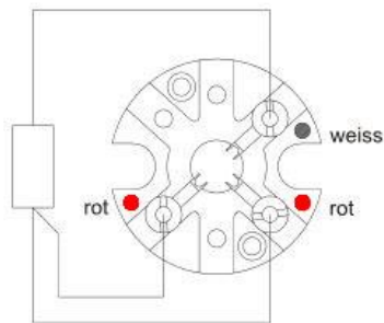
1xPt100 3-Leiter
