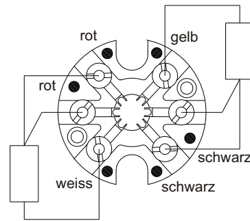
2xPt100 3-Leiter
