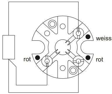
1xPt100 3-Leiter
