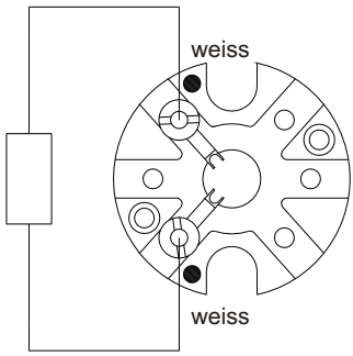
1xPt100 2-Leiter
