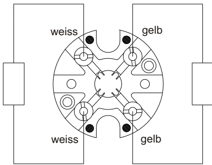
2xPt100 2-Leiter
