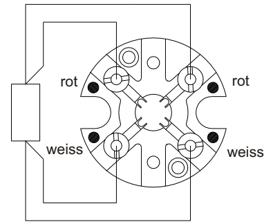
1xPt100 4-Leiter
