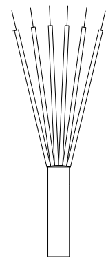
2xPt100
