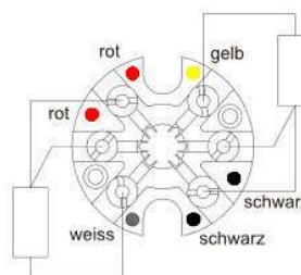
2xPt100 3-Leiter
